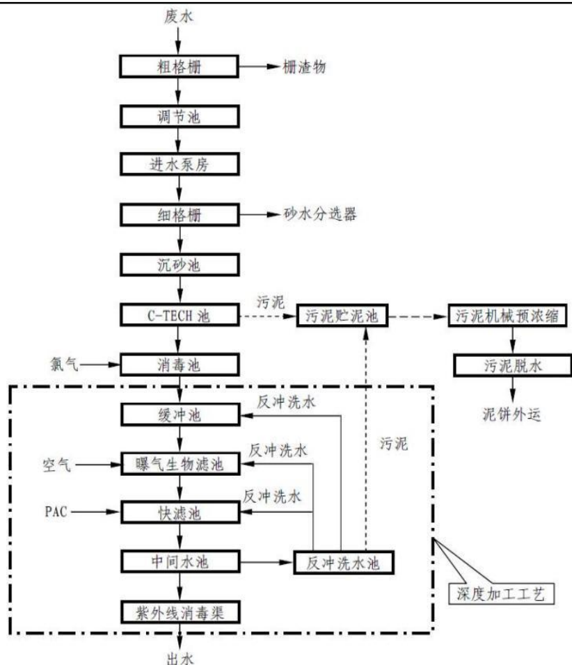
图4-3 城东污水处理厂污水处理工艺流程图
