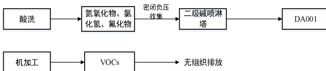
图 4.1-1 废气收集处理示意图
