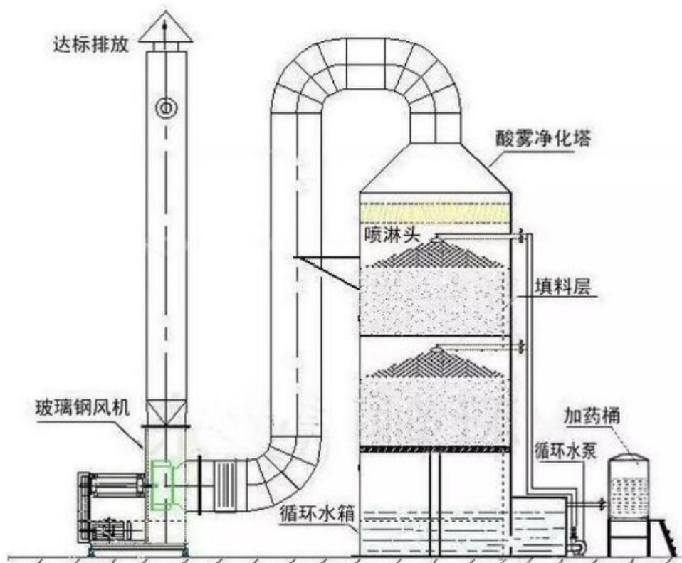
图 4.1-2 碱液喷淋塔结构图
