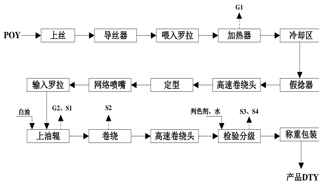
图 5-1 涤纶加弹丝生产工艺流程
