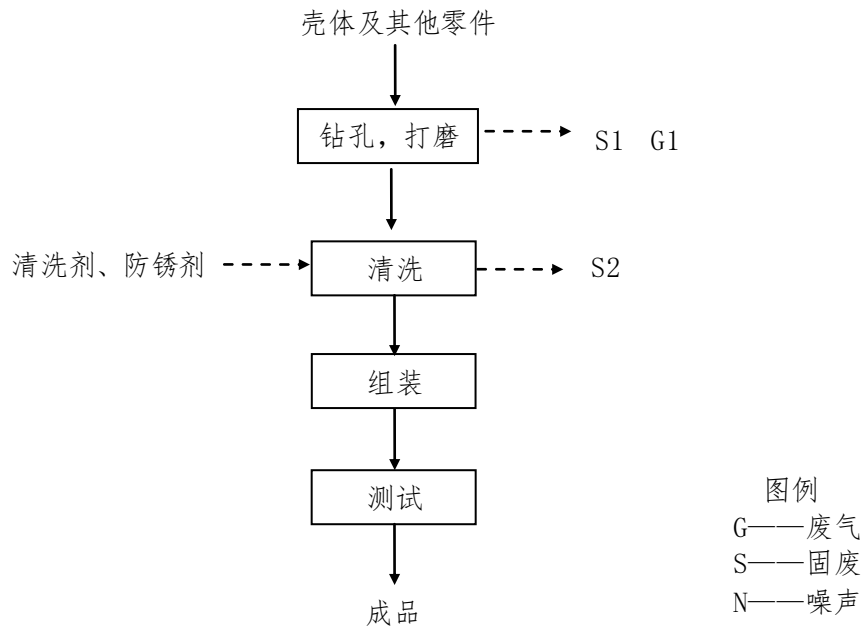
图 1 螺杆式空气压缩机主机生产工艺流程图
