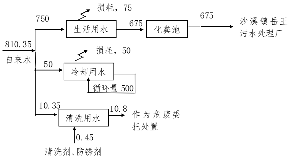
图 2 建设项目完成后全厂用排水平衡图 (单位 t/a)
