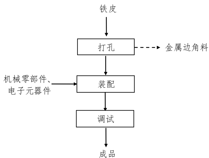
图1 自动粪便分析仪生产工艺流程图
