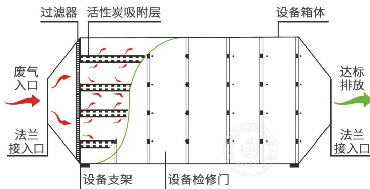
图 4-3 活性炭箱结构示意图及工作原理
