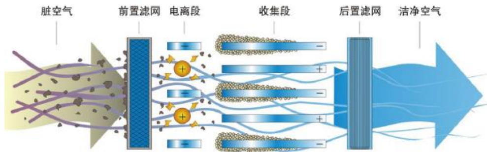
图 4-2 静电油烟装置结构示意图及工作原理
