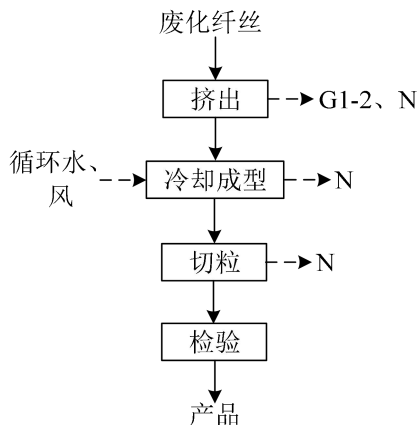
图 2-3 工艺流程及产污环节图
