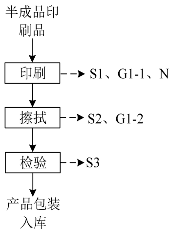
图2-1 印刷品生产工艺流程及产污环节图
