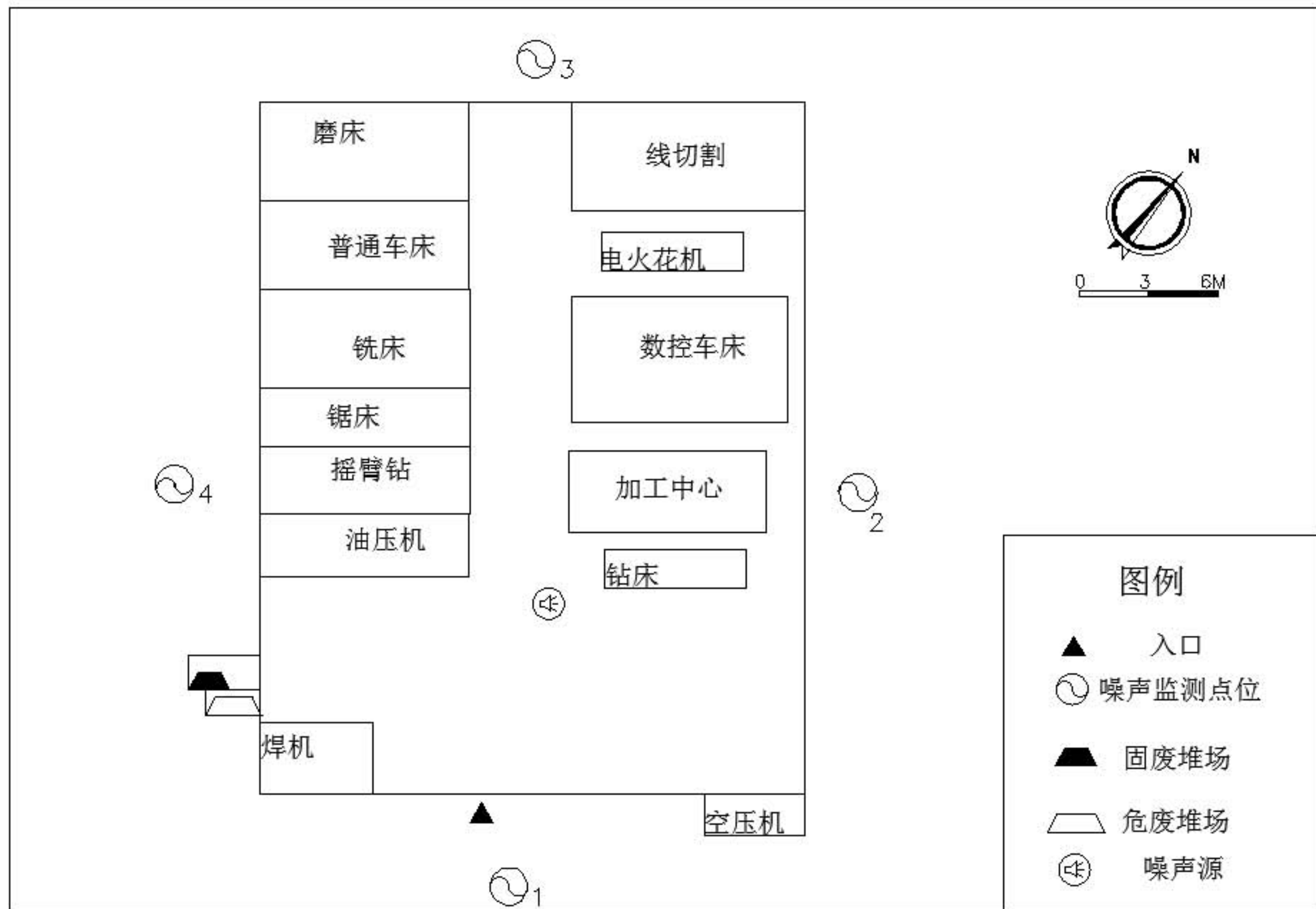
附图三 建设项目平面布置图
