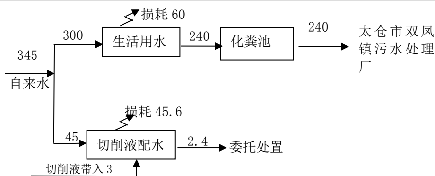
图 4 建设项目全厂用排水平衡图 （单位 t/a）
