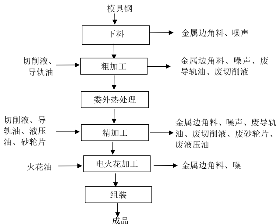
图 2 模具生产工艺流程图
