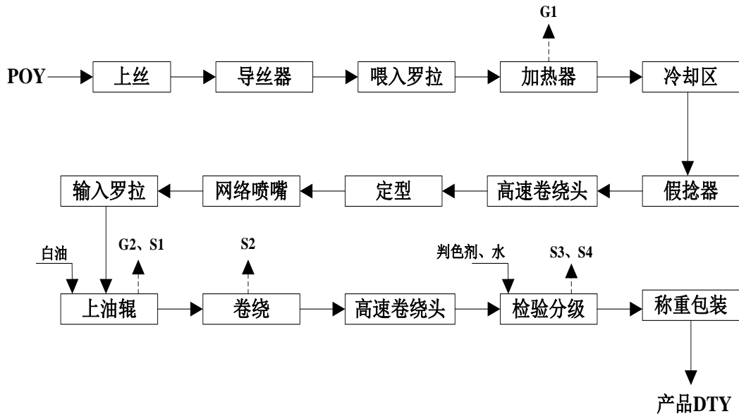
图 5-1 化纤丝生产工艺流程
