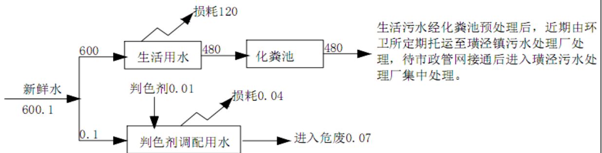
图 5-2 本项目水平衡图 (t/a)
