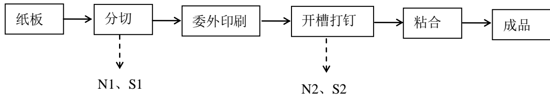
图 5-1 纸箱生产工艺流程及产污节点图
