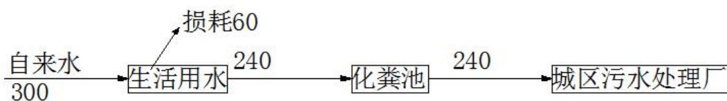
图 5-2 项目水平衡图
