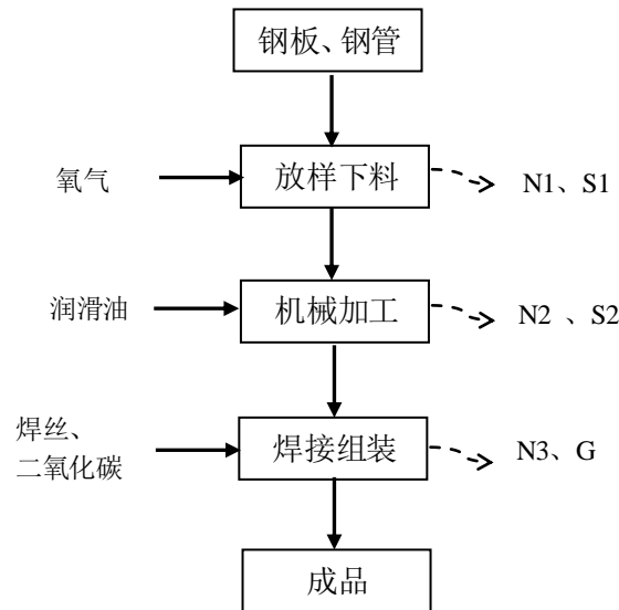
图 5-1 建设项目生产工艺流程图
