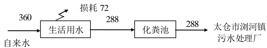
图 5-3 建设项目用排水平衡图（单位 t/a）
