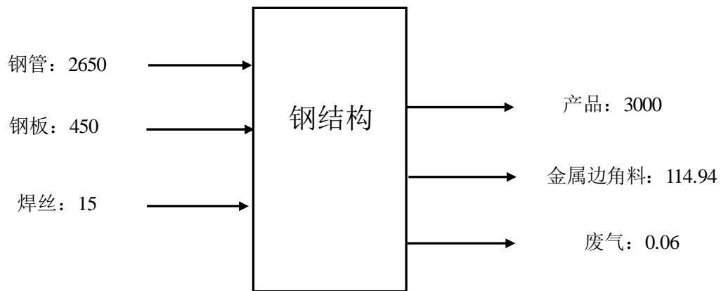
图 5-2 建设项目物料平衡图 (单位: t/a)
