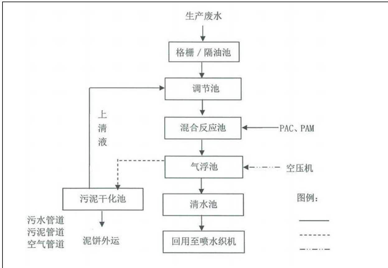
图 7-1 污水处理工艺流程图
