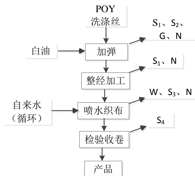
图 5-1 本项目生产工艺及产污环节图
