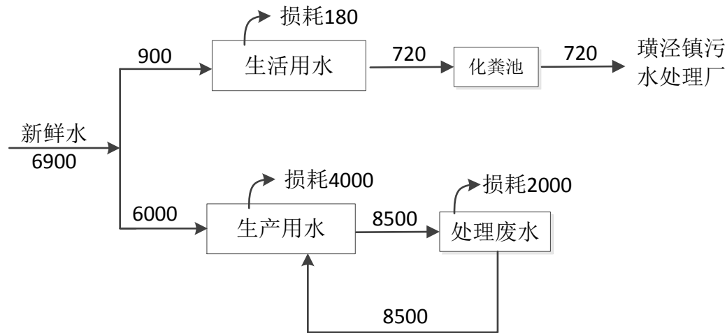
图 5-3 项目水平衡图 单位： t/a
