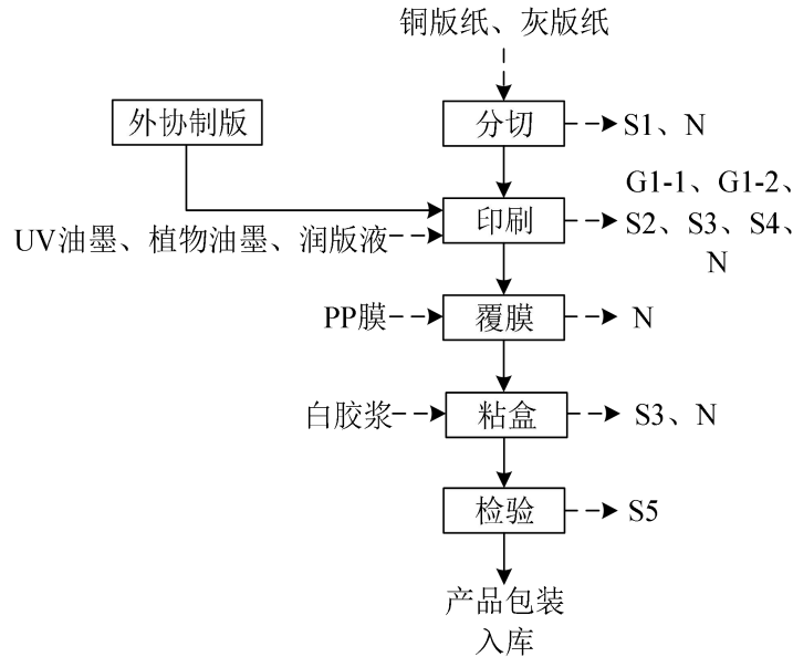
图 5-3 盒子印刷工艺流程及产污环节图
