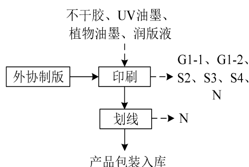
图 5-4 不干胶印刷工艺流程及产污环节图
