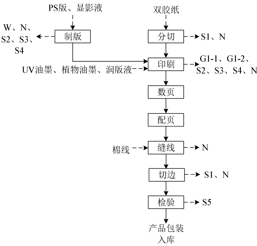
图 5-1 作业本印刷工艺流程及产污环节图
