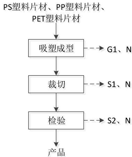
图2-1 塑料包装盒生产工艺流程及产污环节图
