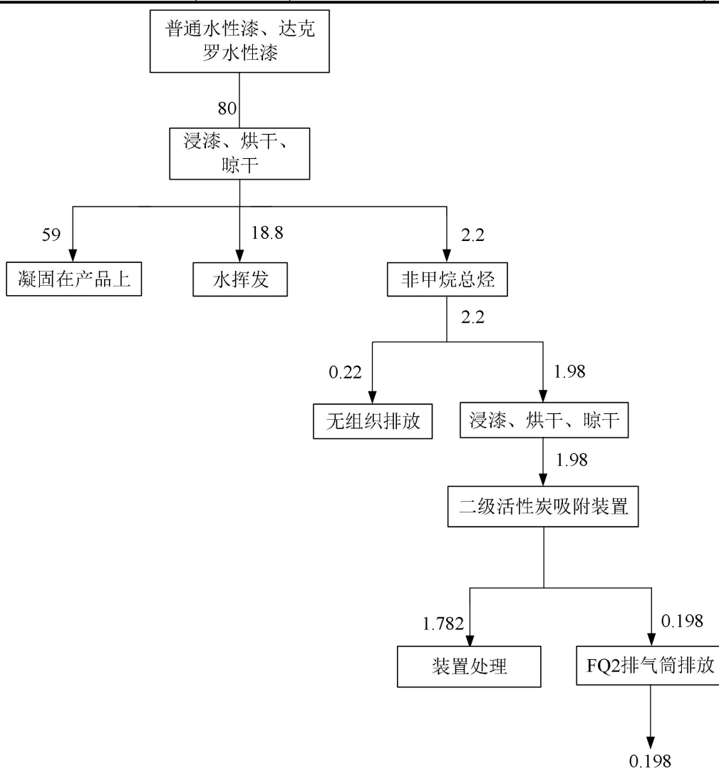
图 4-1 本项目物料平衡图 (t/a)
