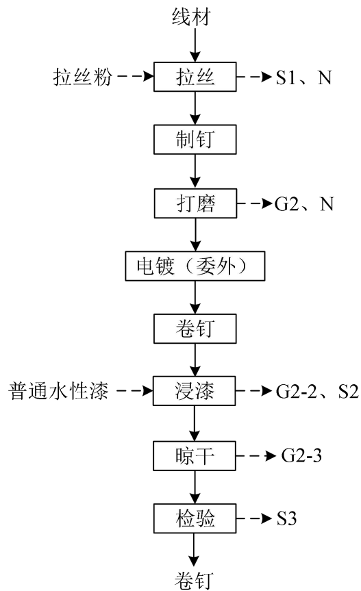
图 2-2 卷钉生产工艺及产污环节图
