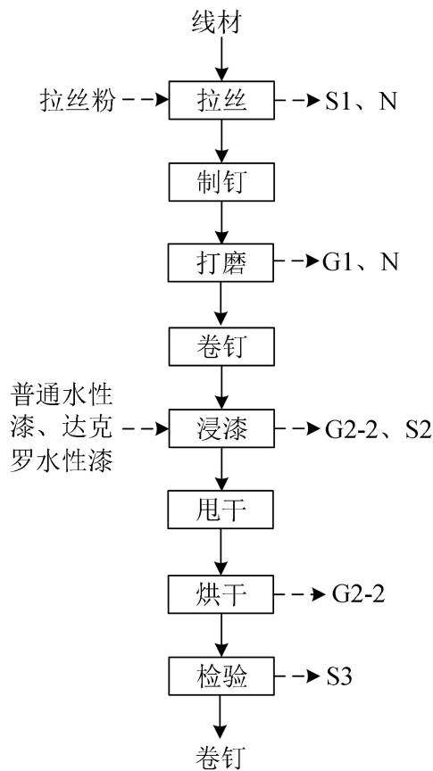
图 2-1 卷钉生产工艺及产污环节图
