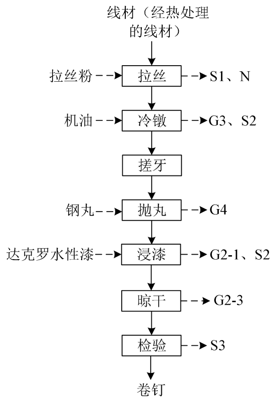
图 2-4 螺丝生产工艺及产污环节图
