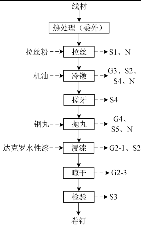
图 2-3 螺丝生产工艺及产污环节图
