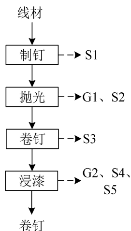
图 2-5 现有项目生产工艺及产污环节图
