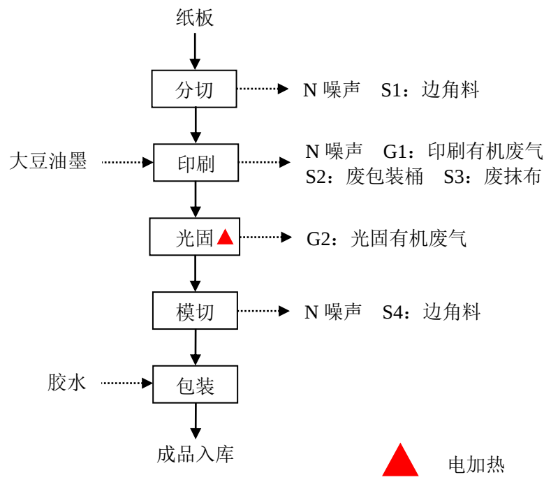
图 5-1 生产工艺流程及产污环节图
