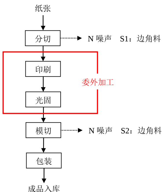
图 1-1 现有项目产品生产工艺流程图
