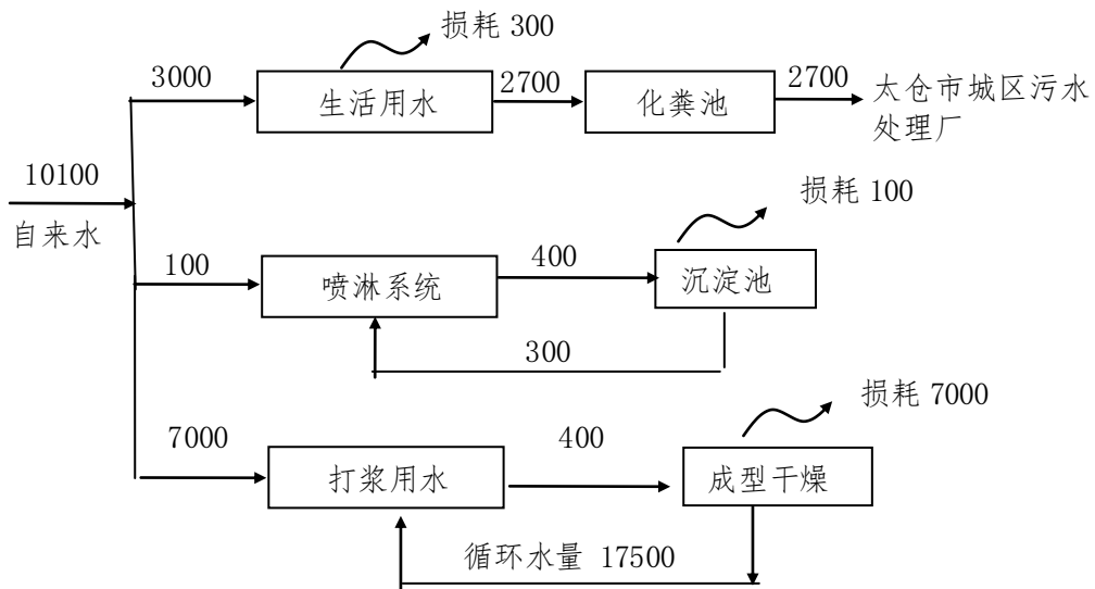
图 6 技改项目全厂用排水平衡图 (t/a)
