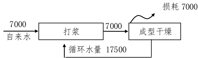
图 5 技改项目用排水平衡图 (t/a)
