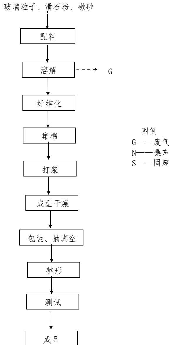
图 2 玻璃棉制品、节能保温材料生产工艺流程
