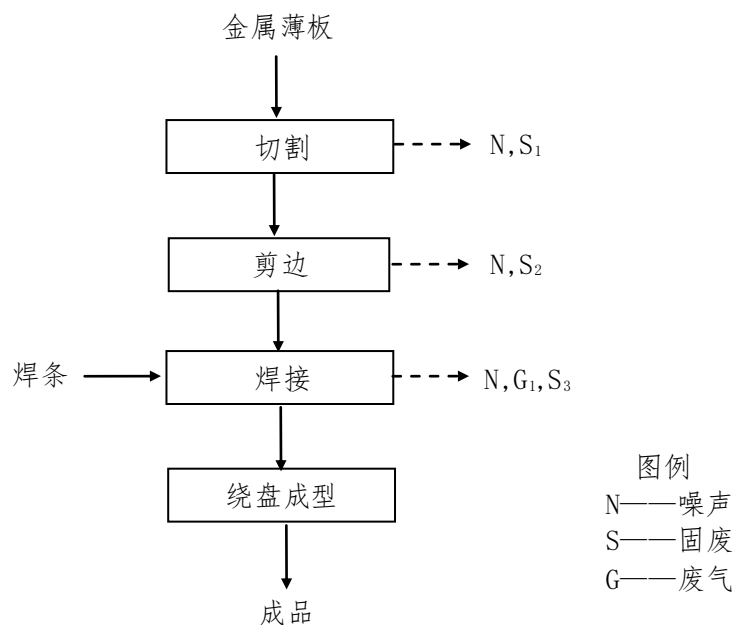
图1 建设项目生产工艺流程图
