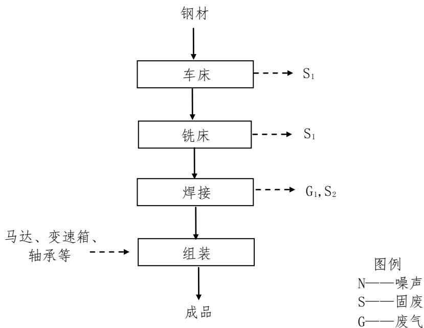
图 1 建设项目生产工艺流程图
