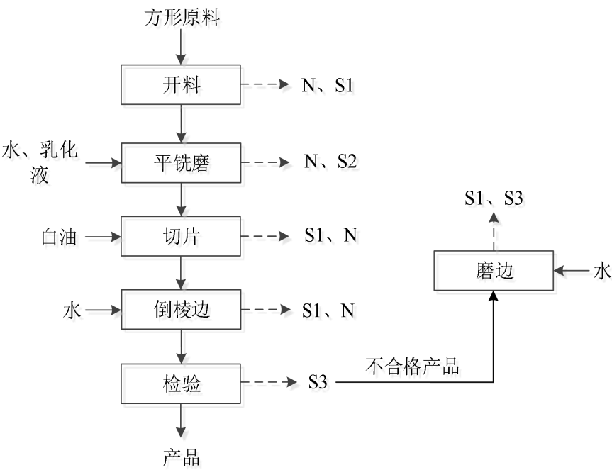
图 5-1 生产工艺流程及产污环节图
