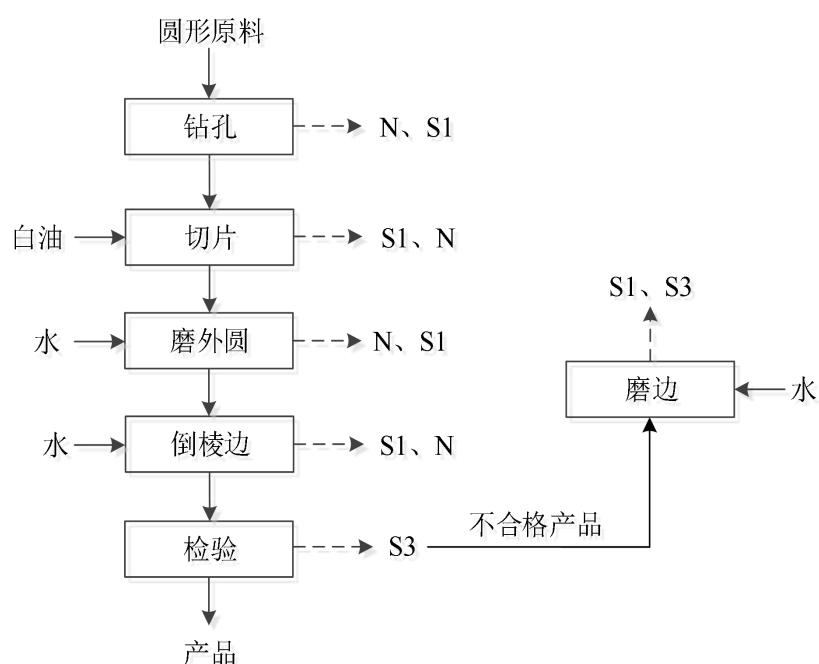
图 5-2 生产工艺流程及产污环节图
