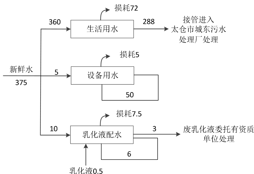
图 5-3 项目水平衡图 (t/a)
