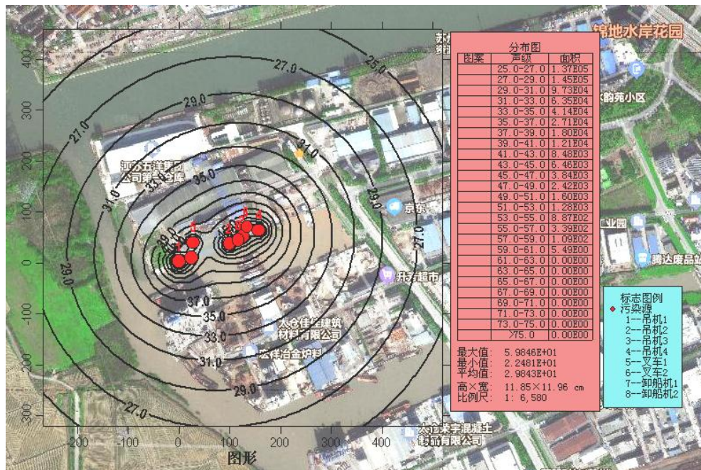
图 4-3 等声级线图
