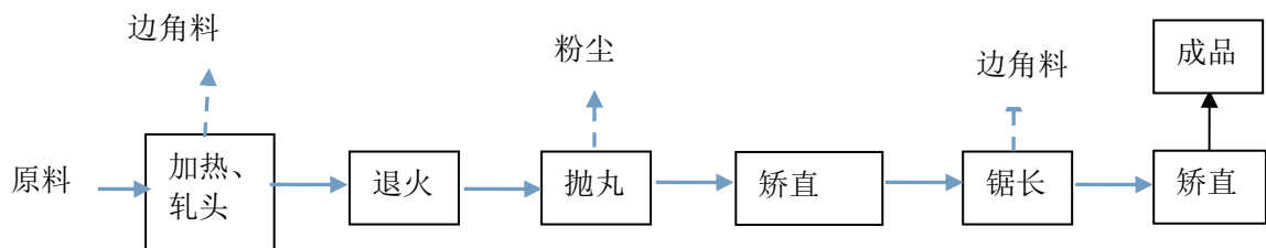
图 1 生产工艺流程
