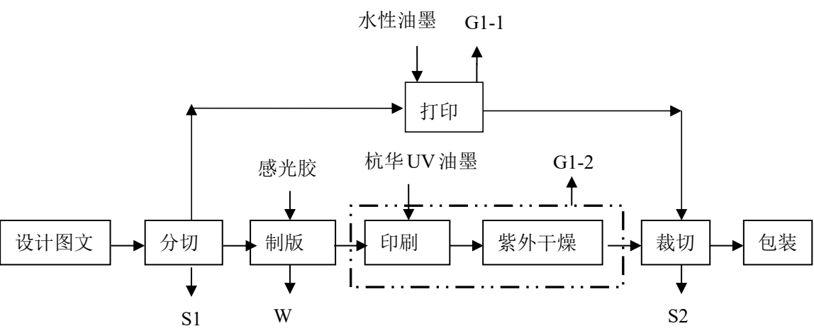
图 5-1 生产工艺流程及产污环节图
