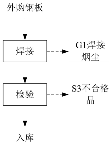
图 2-5 材料熨平底板生产工艺流程图
