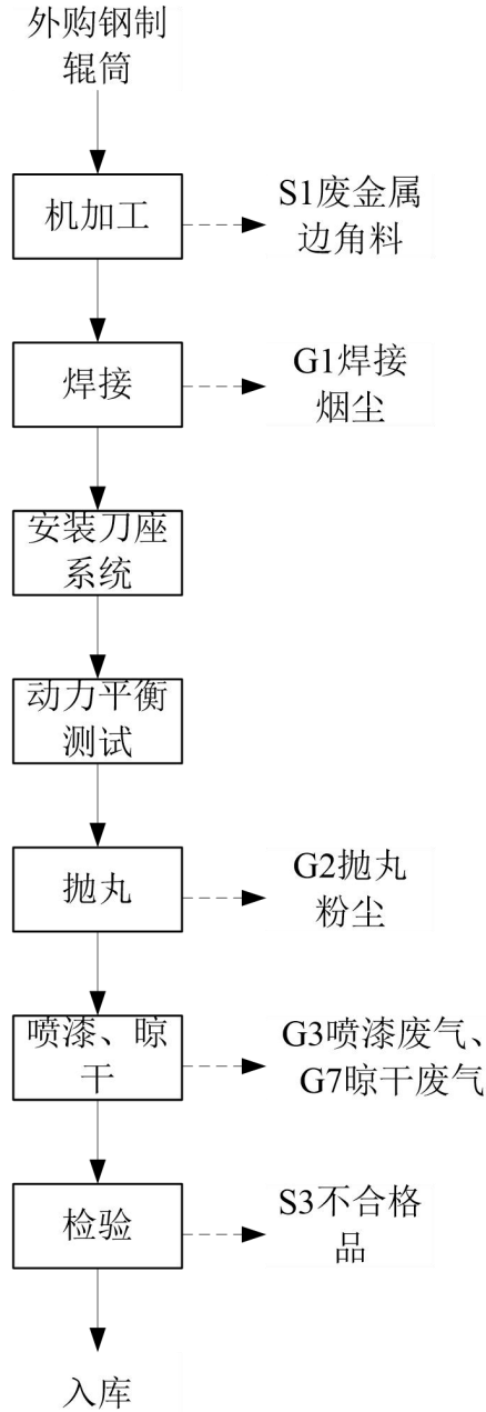
图 2-2 铁芯生产工艺流程图
