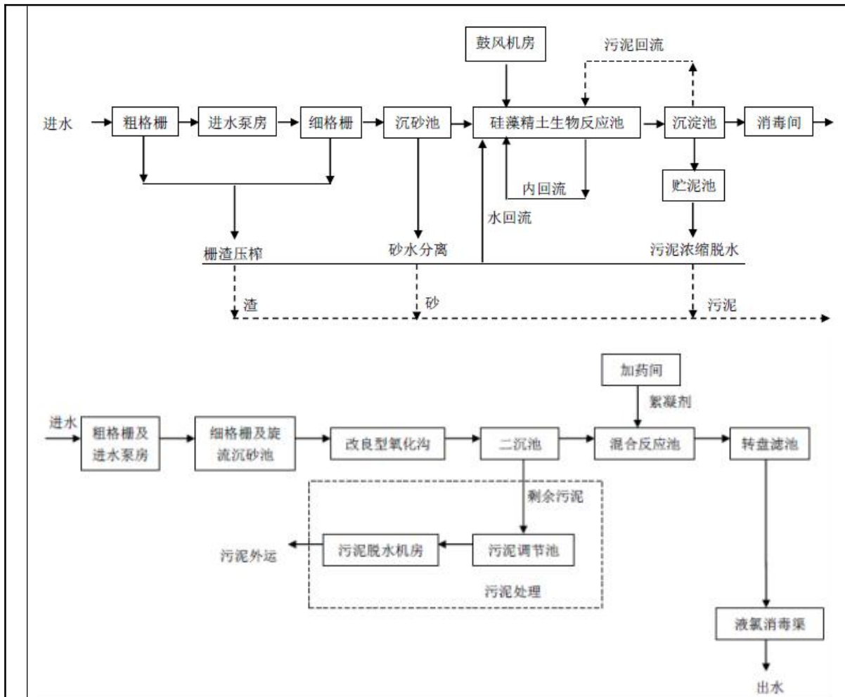
图 4-2 太仓江城城市污水处理有限公司工艺流程图 (上：一期第一阶段，下：一期第二阶段)
