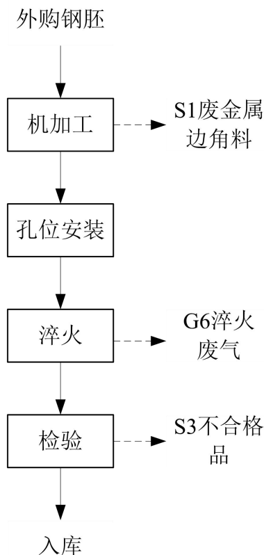
图 2-4 材料夯实压力梁生产工艺流程图
