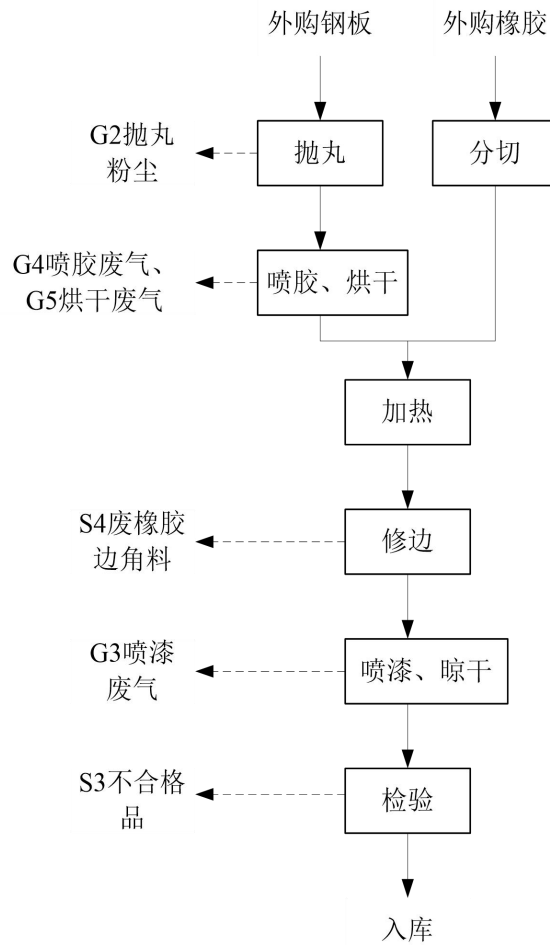
图 2-3 履带部件生产工艺流程图
