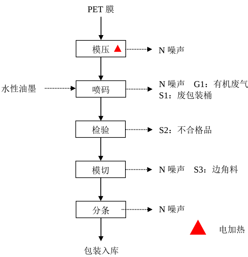
图 5-1 汽车零部件生产工艺流程及产污环节图
