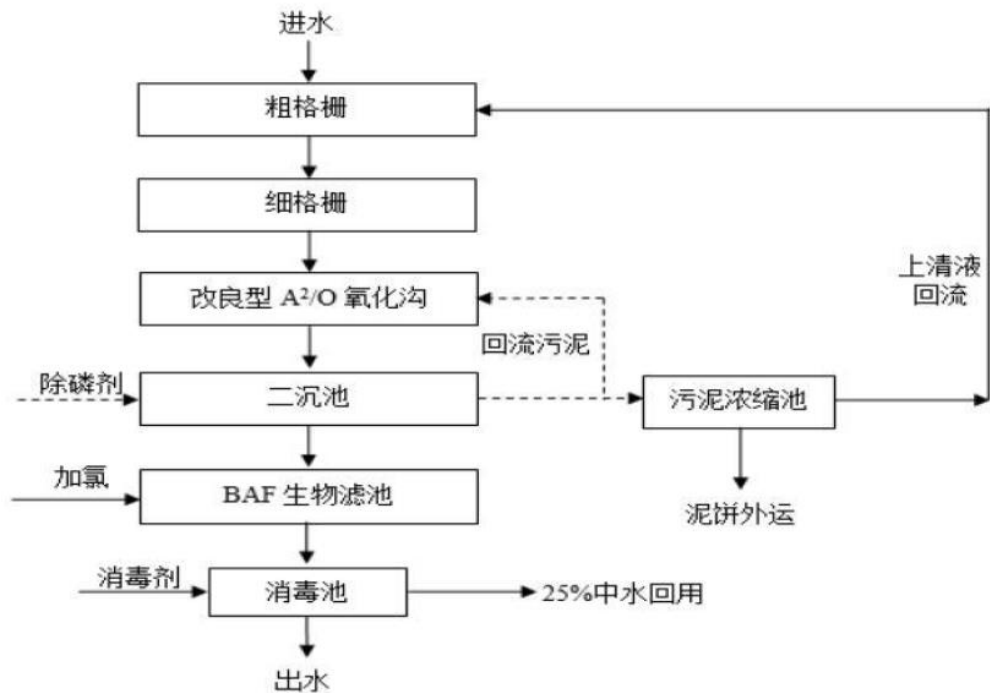
图 7-2 城区污水处理厂污水处理工艺流程图
