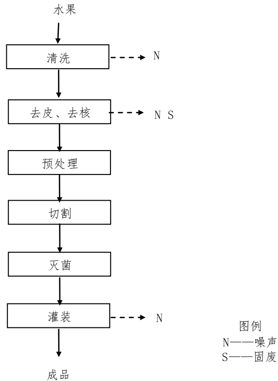
图 1 鲜果粒制品生产工艺流程图
