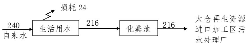
图 2 建设项目用排水平衡图 (单位 t/a)
