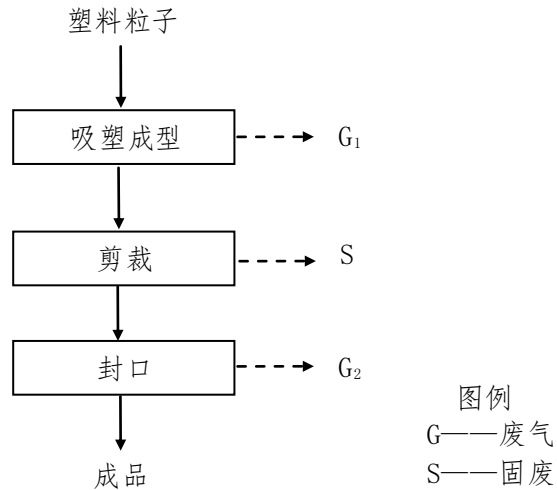
图 1 生产工艺流程图
