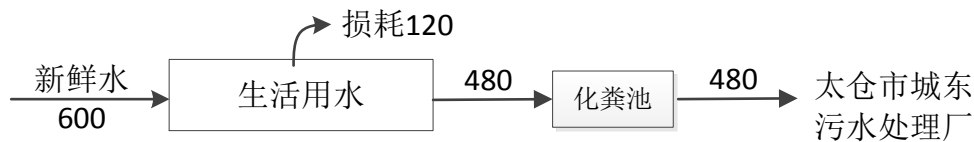
图 5-2 项目水平衡图 t/a
