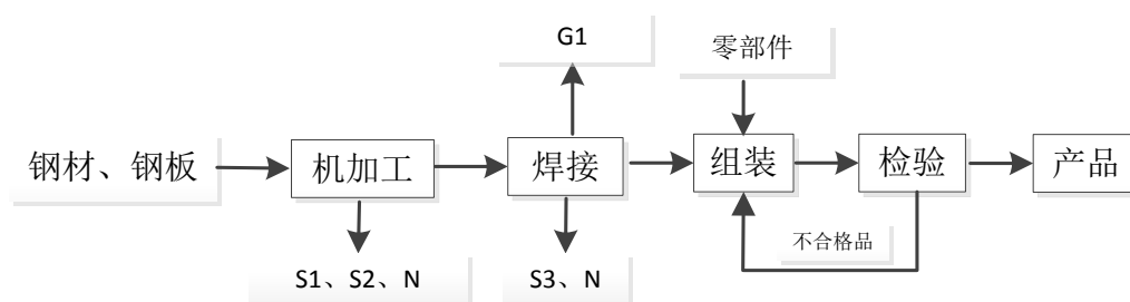
图 5-1 环保设备生产工艺及产污环节图
