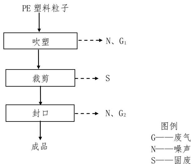
图 1 塑料制品生产工艺流程图
