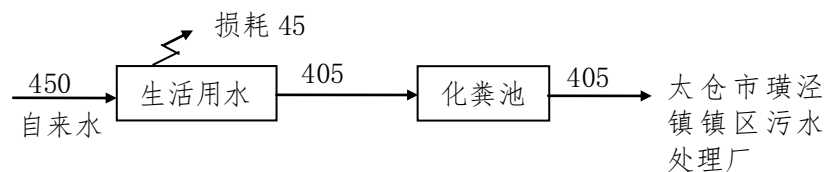
图 2 建设项目全厂用排水平衡图 (单位 t/a)
