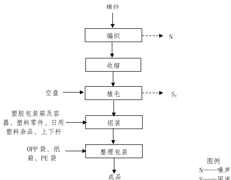
图4 日用清扫工具拖把生产工艺流程图
