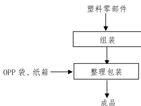
图 1 塑胶包装箱及容器、塑料零件、日用塑料杂品生产工艺流程图
