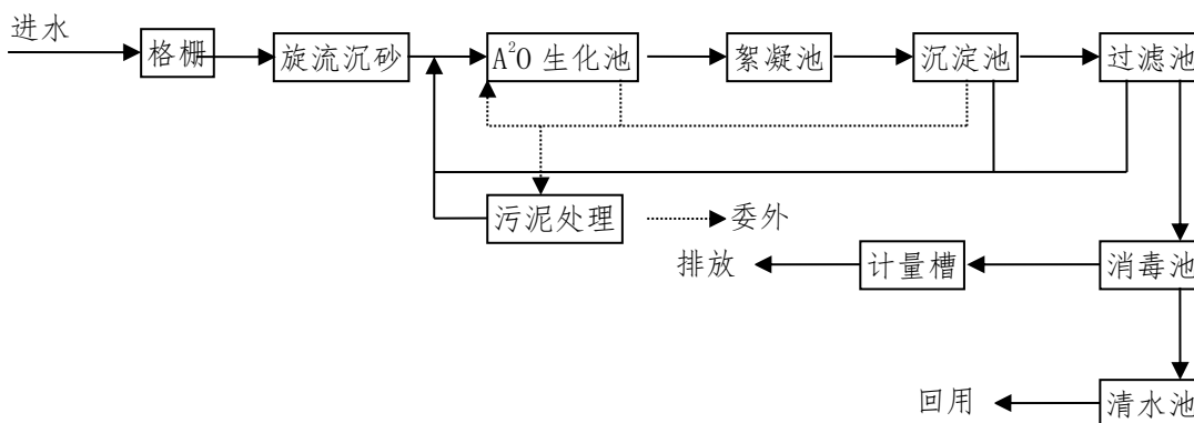
图 6 岳王污水厂的处理流程图
