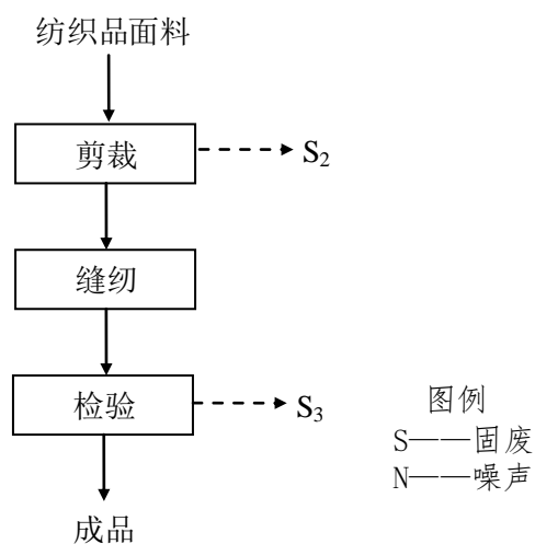
图2 家用纺织品生产工艺流程图
