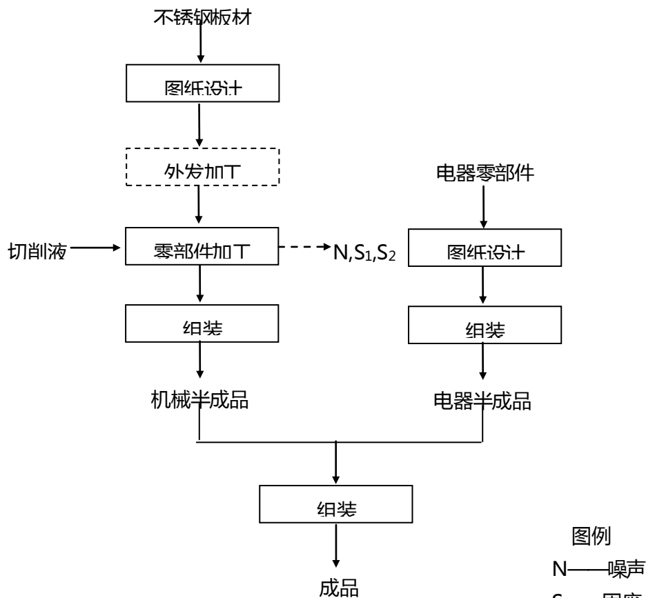
图 1 建设项目生产工艺流程图
