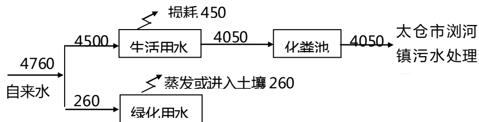
图 2 建设项目用排水平衡图（单位 t/a）
