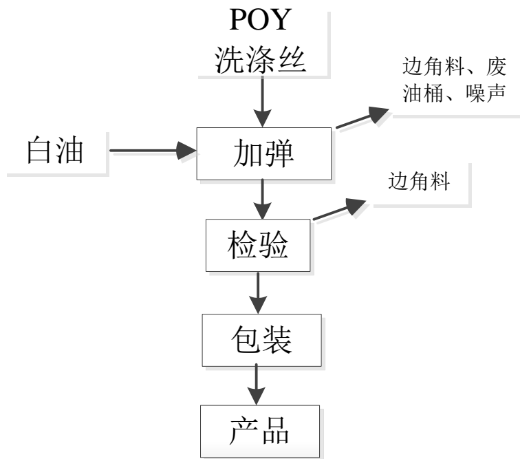
图 1-1 化纤加弹丝生产工艺及产污环节图
