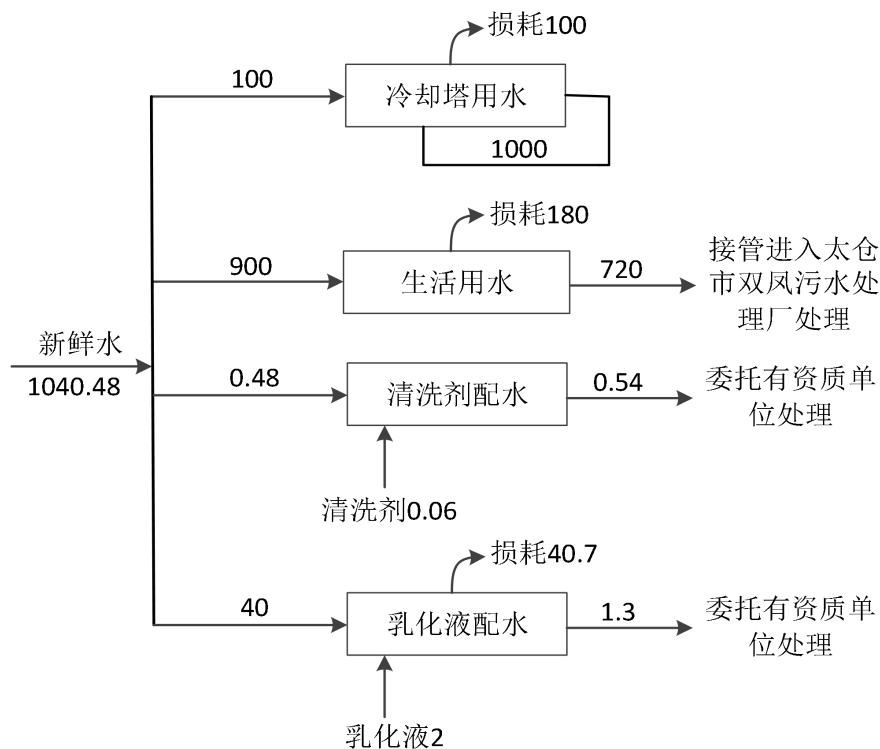
图 5-3 项目水平衡图 (t/a)
