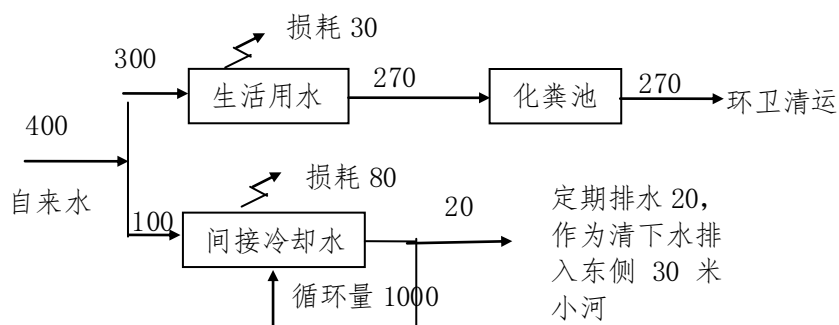
图2 建设项目用排水平衡图 (单位 t/a)
