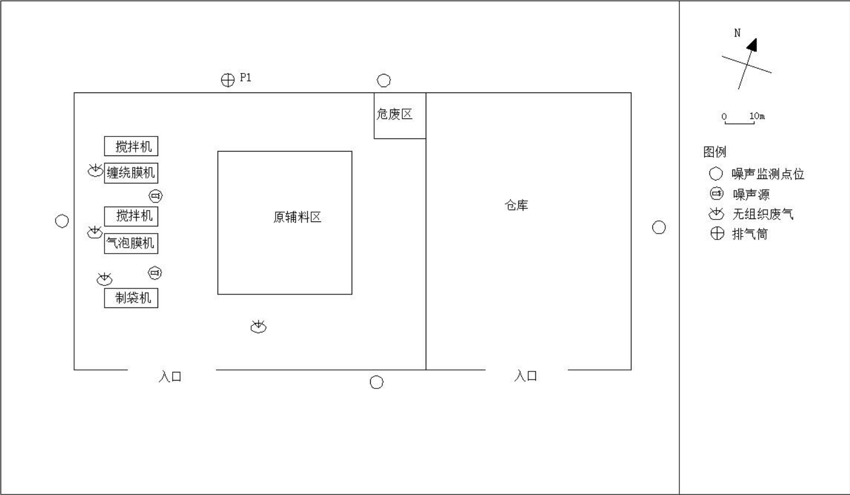
附图三 建设项目厂区平面布置图
