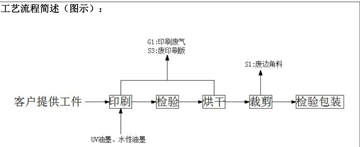
图 5-1 工艺流程及产污环节图
