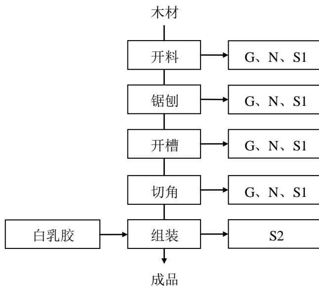
图 5-1 生产工艺流程及产污节点图
