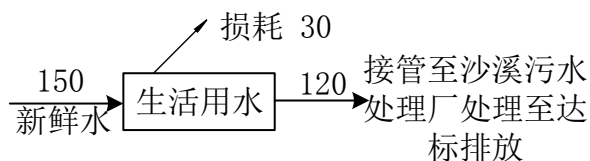
图 1-2 原有项目水平衡图 单位: t/a
