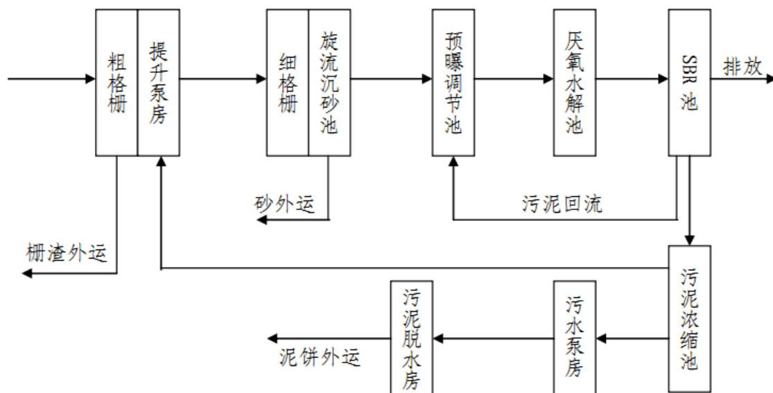
图 7-2 太仓市沙溪污水处理厂工艺流程图
