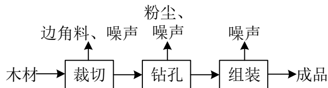
图 1-1 原项目生产工艺流程及产污环节图
