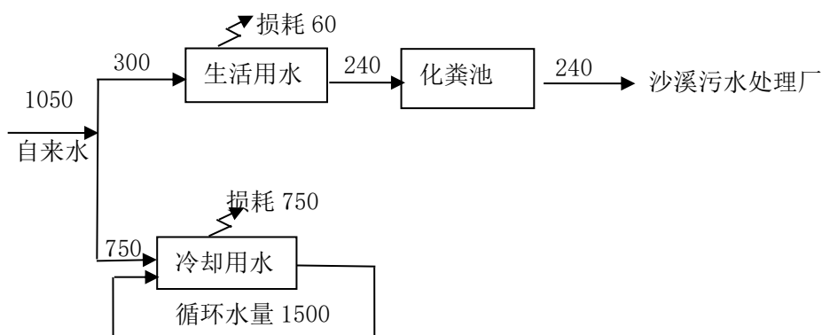
图 2 建设项目全厂用排水平衡图 (单位 t/a)
