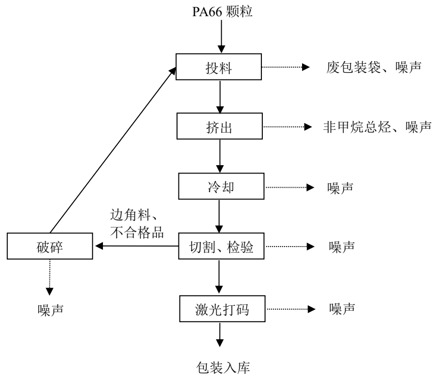
图 1 尼龙隔热条生产工艺流程及产污环节图
