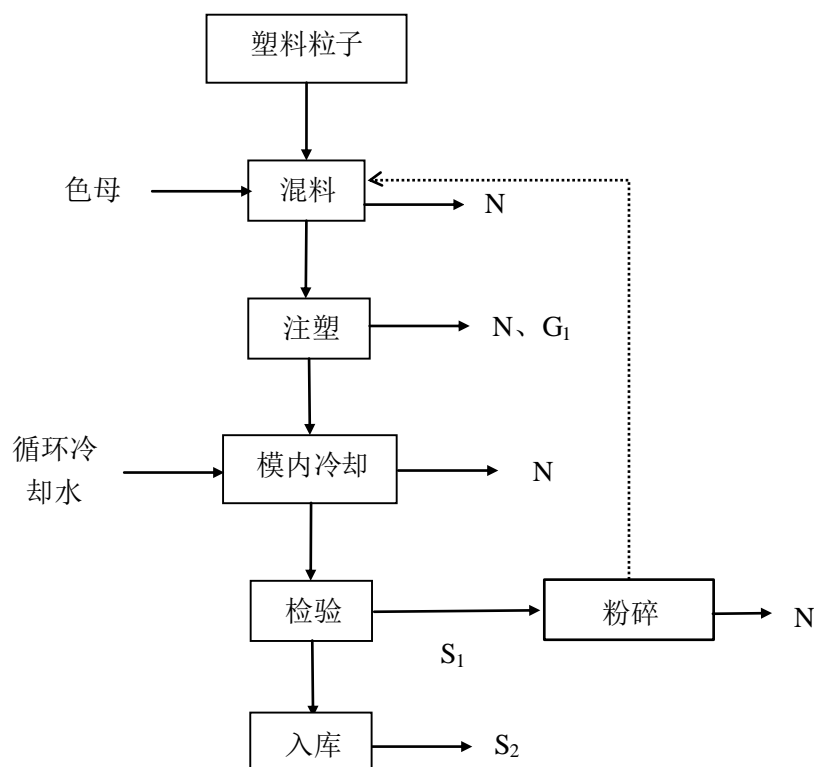
图 5-1 塑料制品生产工艺及产污环节图
