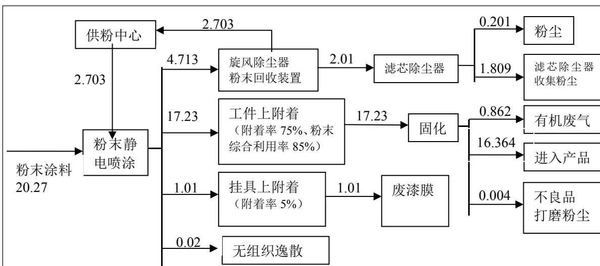
图 5-2 本项目粉末涂层物料平衡图 (t/a)
