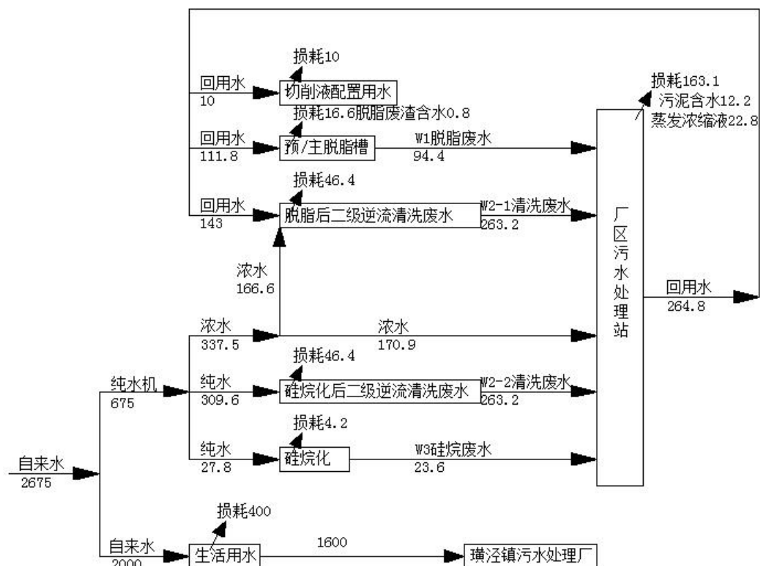
图 5-3 本项目水平衡图 (t/a)
