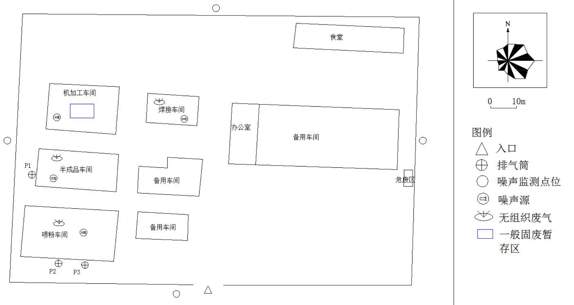
附图三 建设项目厂区平面布置图
