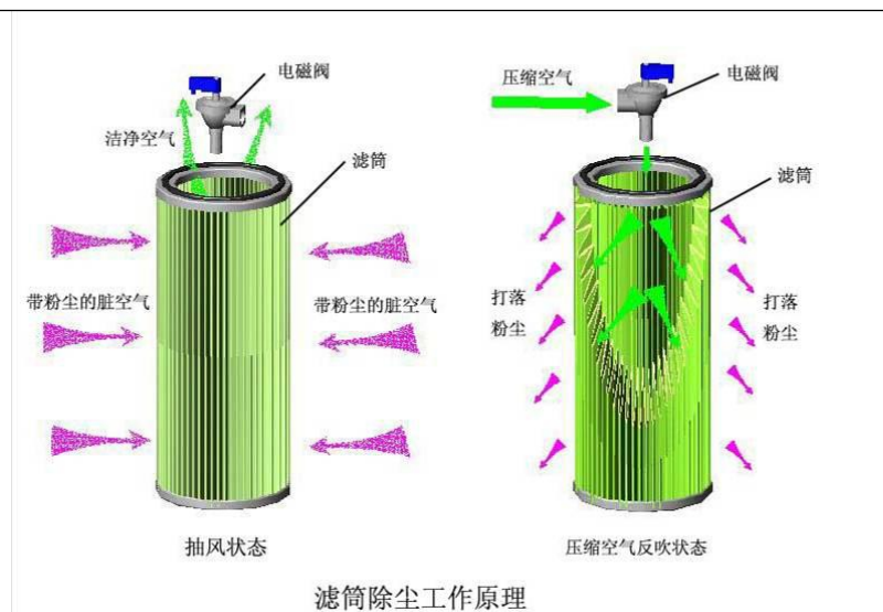
图 7-2 滤筒除尘工作原理图
