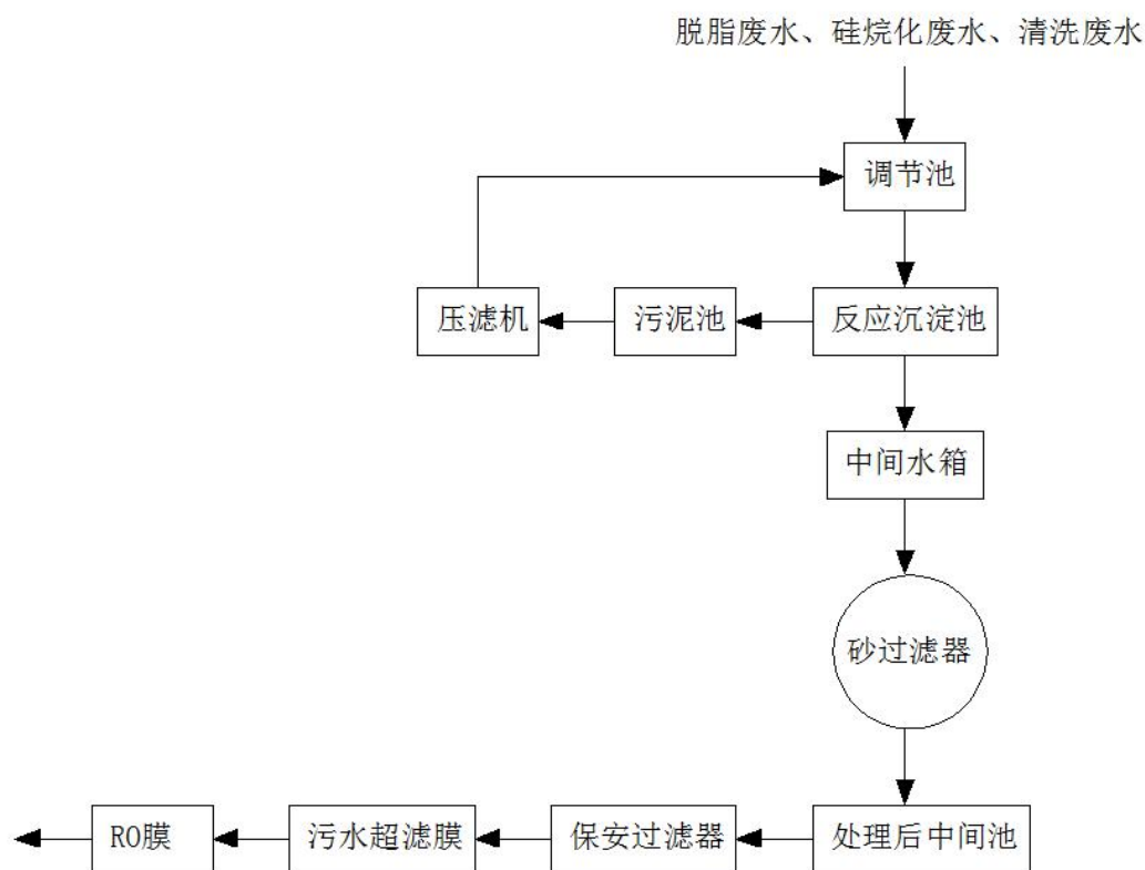
7-5 废水处理工艺流程图
