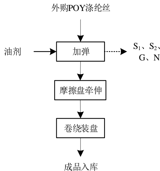
图 1-1 加弹丝生产工艺流程及产污环节图
