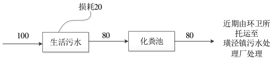
图 1-2 现有项目水平衡图 (t/a)
