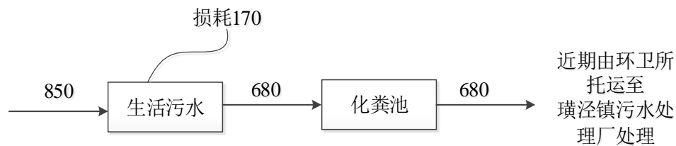
图 5-3 全厂水平衡图 (t/a)
