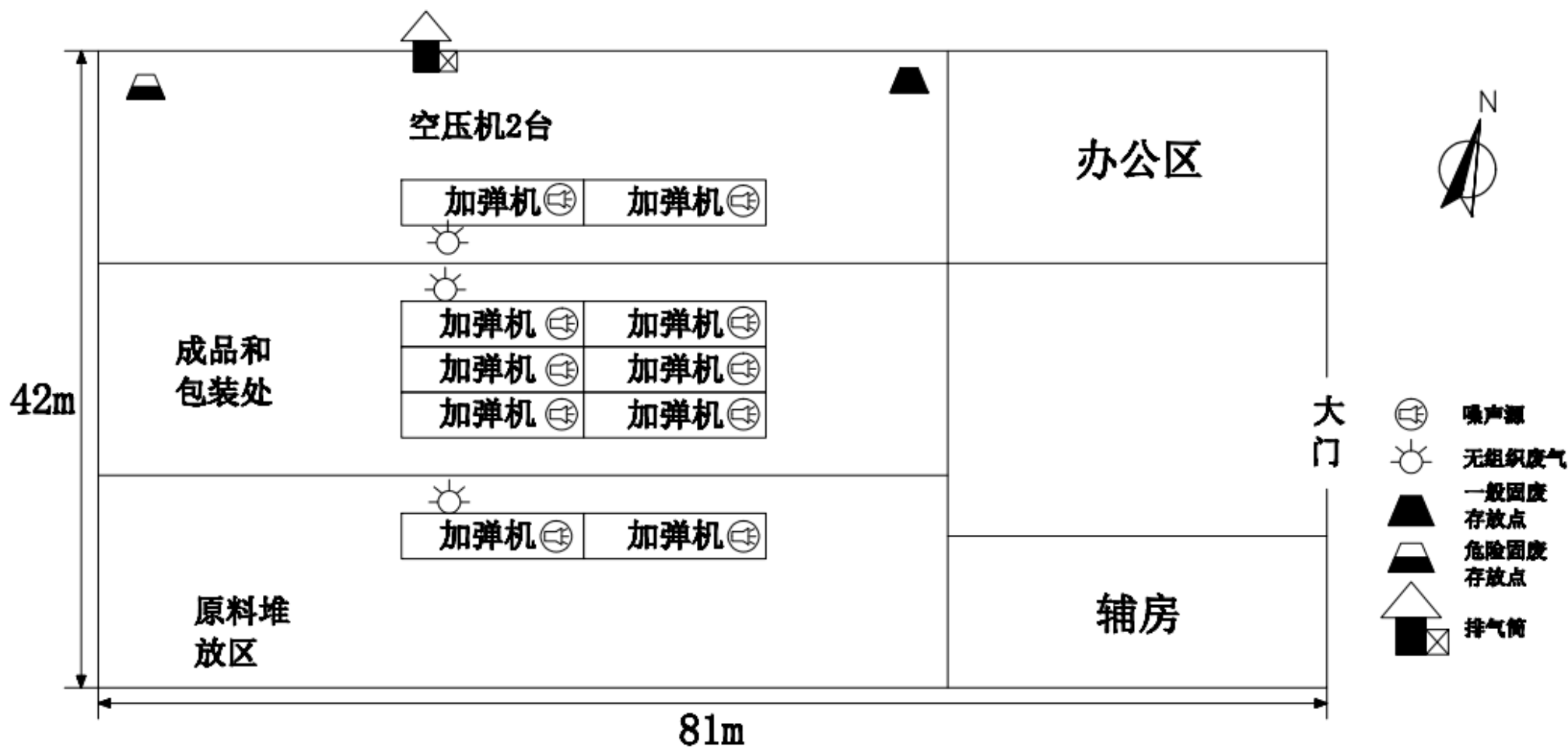
附图 3 项目生产车间平面布置图
