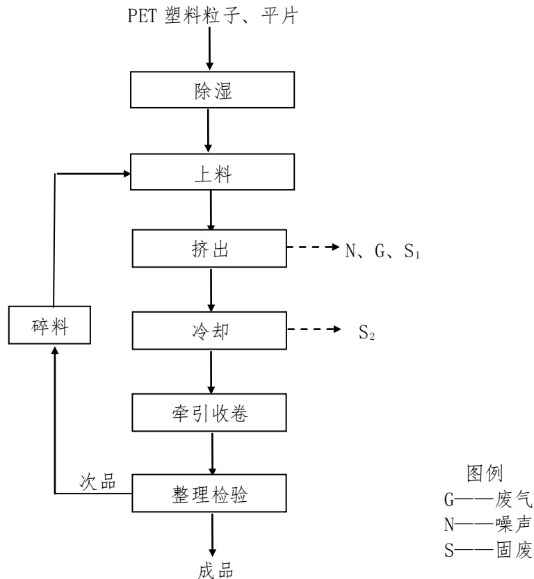
图1 塑钢带生产工艺流程图
