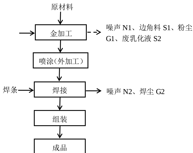
图 5-1 建设项目生产工艺流程图
