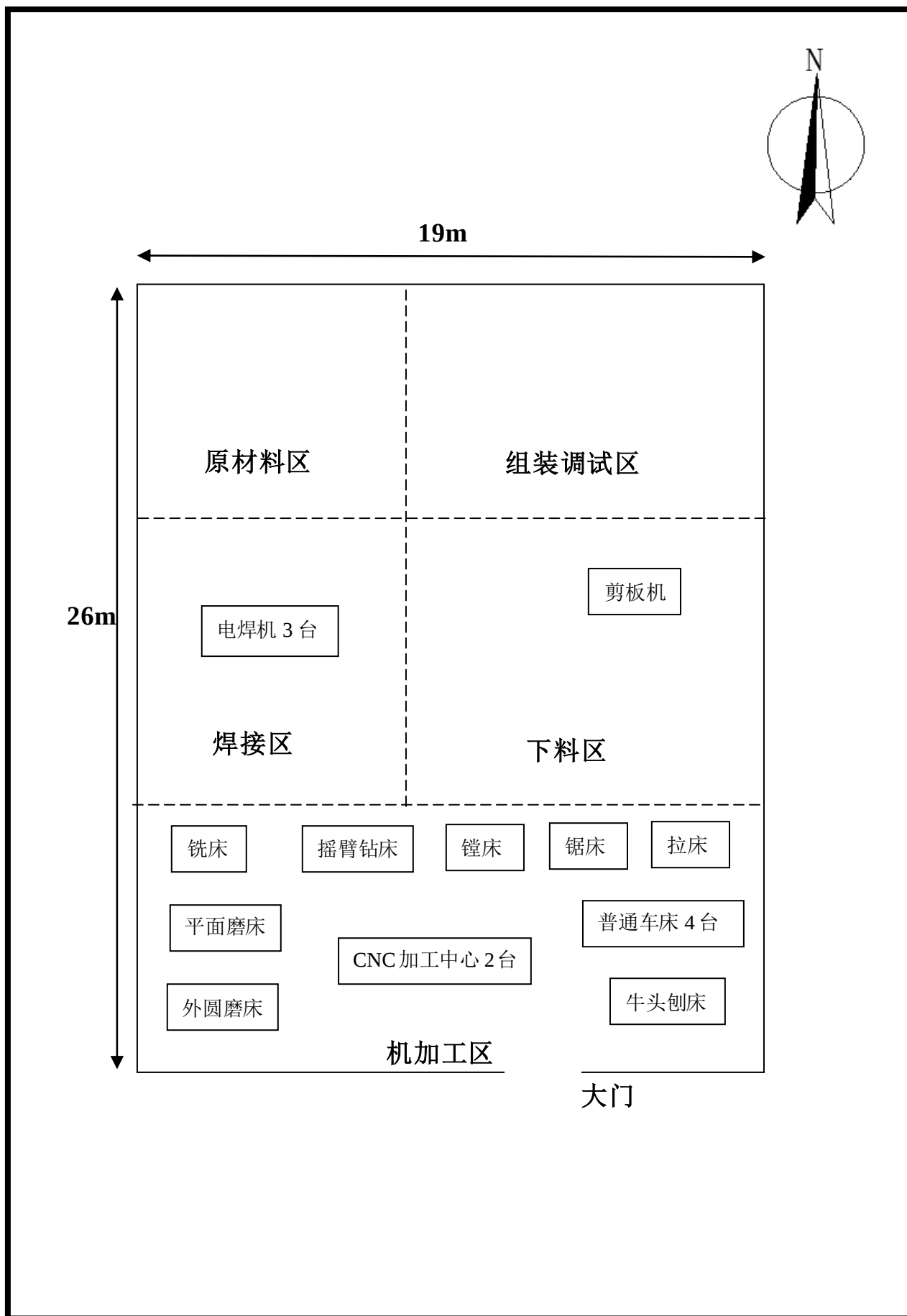
附图 4 车间设备布置图
