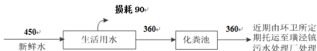
图 5-2 本项目水平衡图 (t/a)
