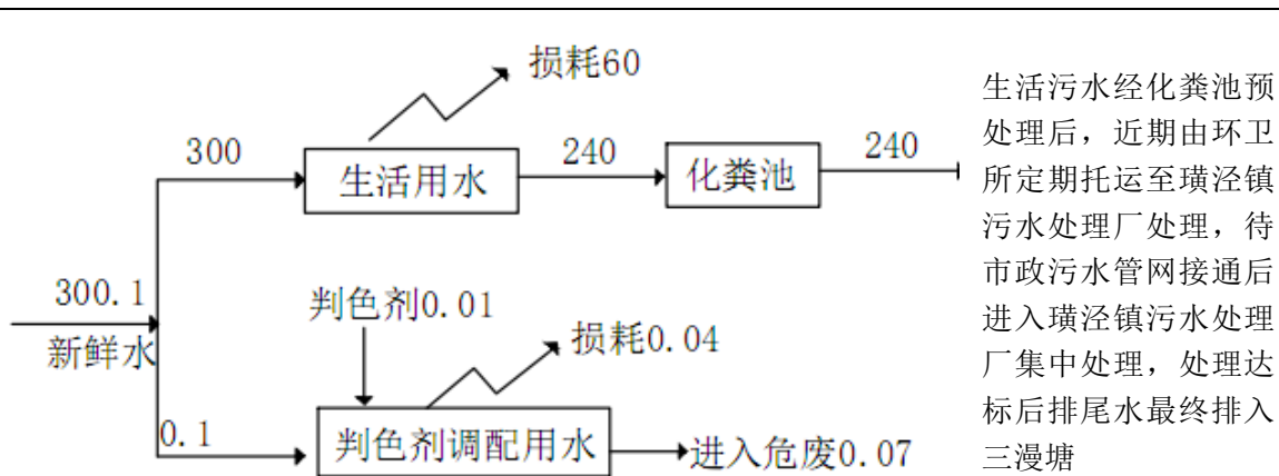
图 5-2 扩建项目水平衡图 (t/a)
