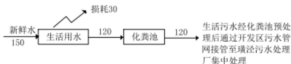
图 1-2 原有项目水平衡图 (t/a)
