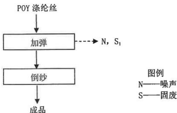
图 2.1-1 涤纶加弹丝生产工艺及产污节点图
