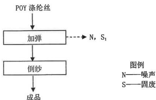
图 3-3 涤纶加弹丝生产工艺及产污节点图
