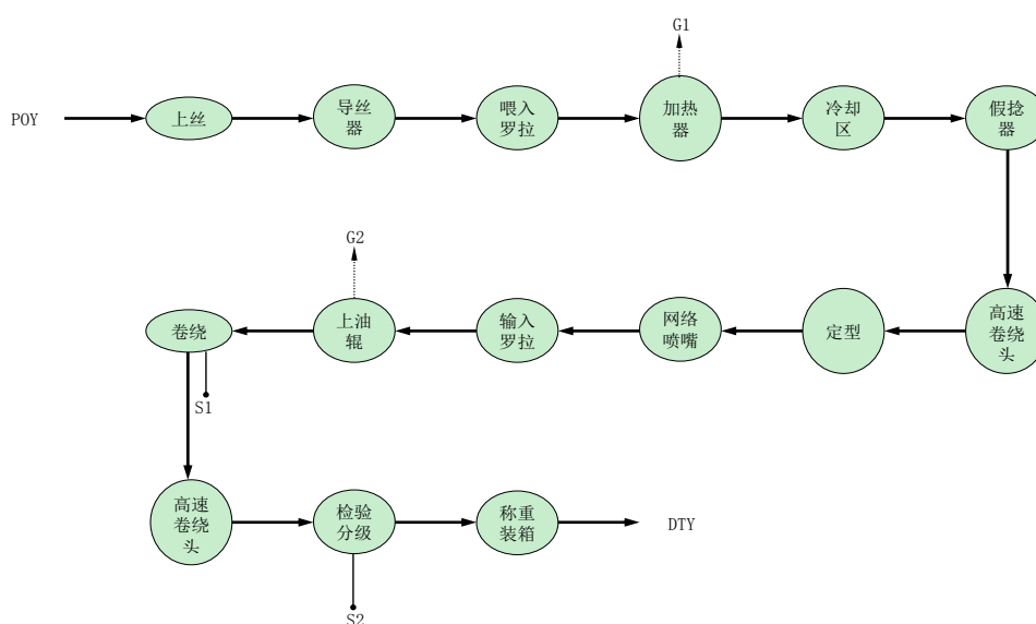
图 1-1 加弹丝生产工艺流程及产污环节图
