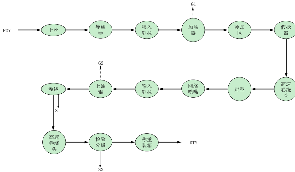
图 5-1 DTY 生产工艺流程
