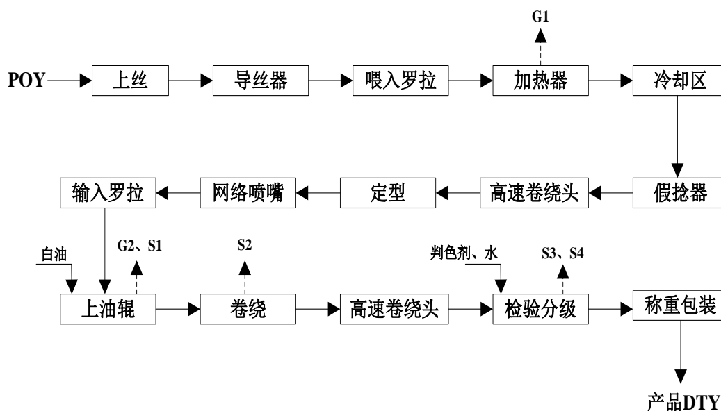
图 5-1 POY 涤纶丝生产工艺流程及产污节点图
