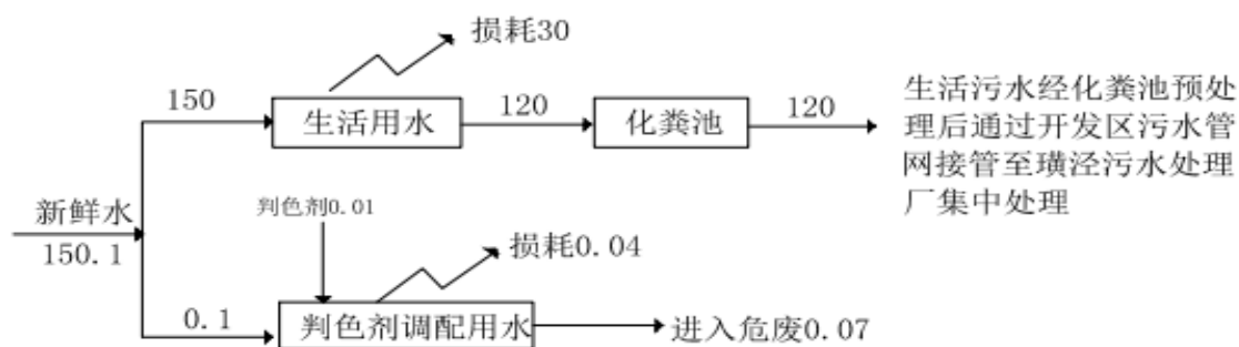
图 5-2 本项目水平衡图 (t/a)
