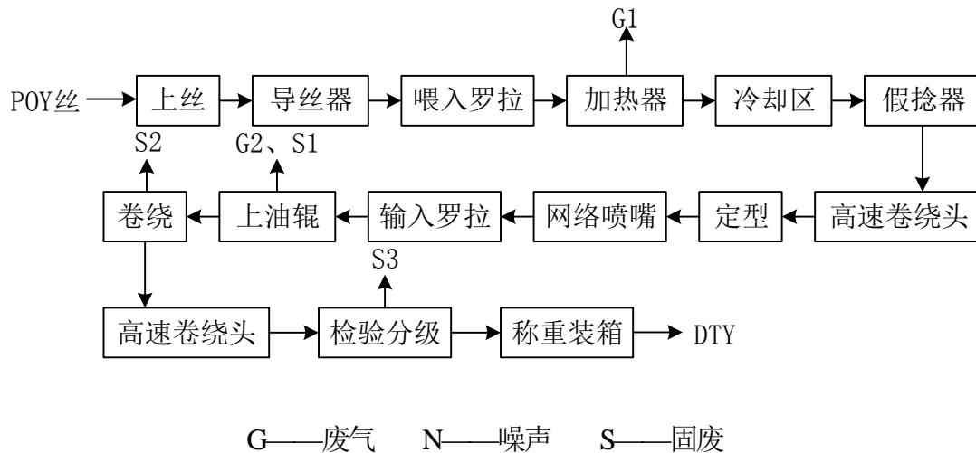
图 5-1 涤纶 DTY 加弹丝生产工艺流程及产污节点图
